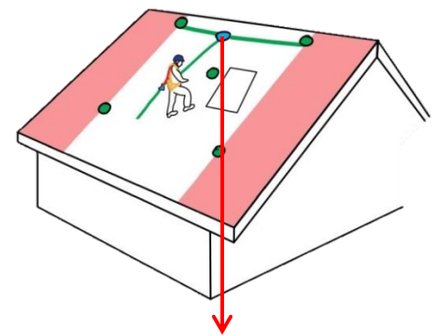
SISTEMA LINEA VITA CONTINUA (2)
