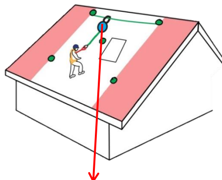
SISTEMA LINEA VITA CONTINUA (1)
