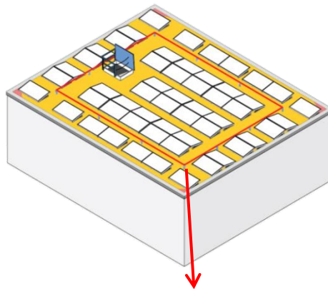
SISTEMA LINEA VITA CONTINUA
