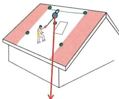
SISTEMA LINEA VITA CONTINUA
